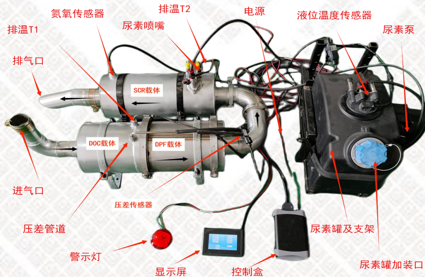
装置图片:
